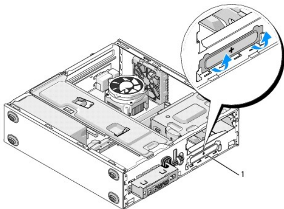
1 3.5 インチベイの取り外し金属プレート
